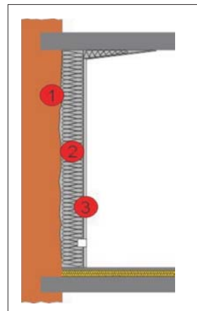
Systematischer Querschnitt der gedämmten Außenwand
